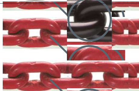
CONDIZIONI DOPO 528 H Si cominciano a vedere i primi segnali di corrosione della vernice. FINAL STATE AFTER 528 H The first signs of corrosion of the paint are noticed.
