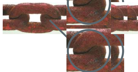
CONDIZIONI DOPO 168 H Precoce deterioramento dello strato protettivo verniciato. FINAL STATE AFTER 168 H Early deterioration of the protective paint layer.
